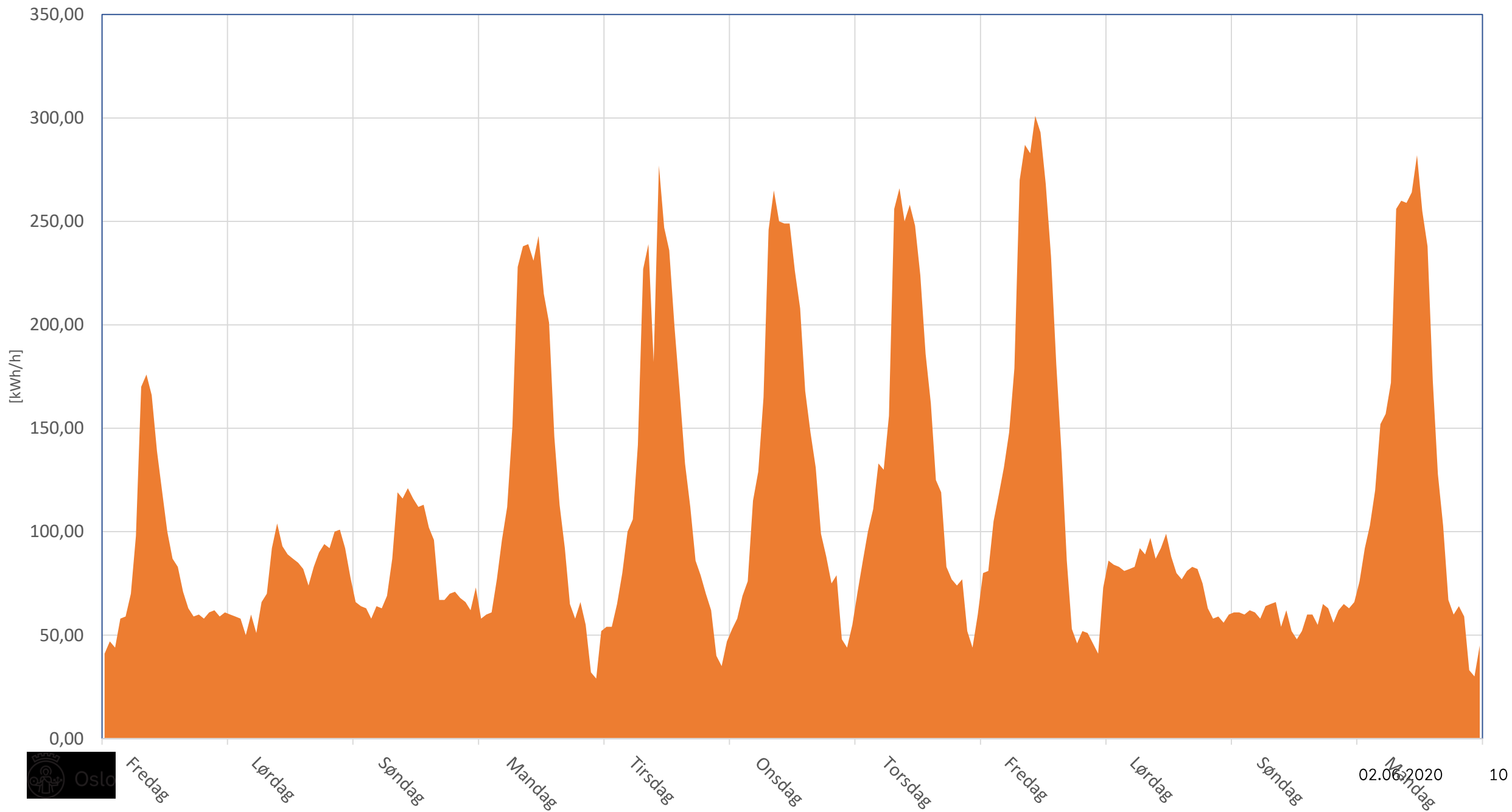
Nordseter ungdomsskole – energiforbruk 11 dager i oktober, før rehabilitering
