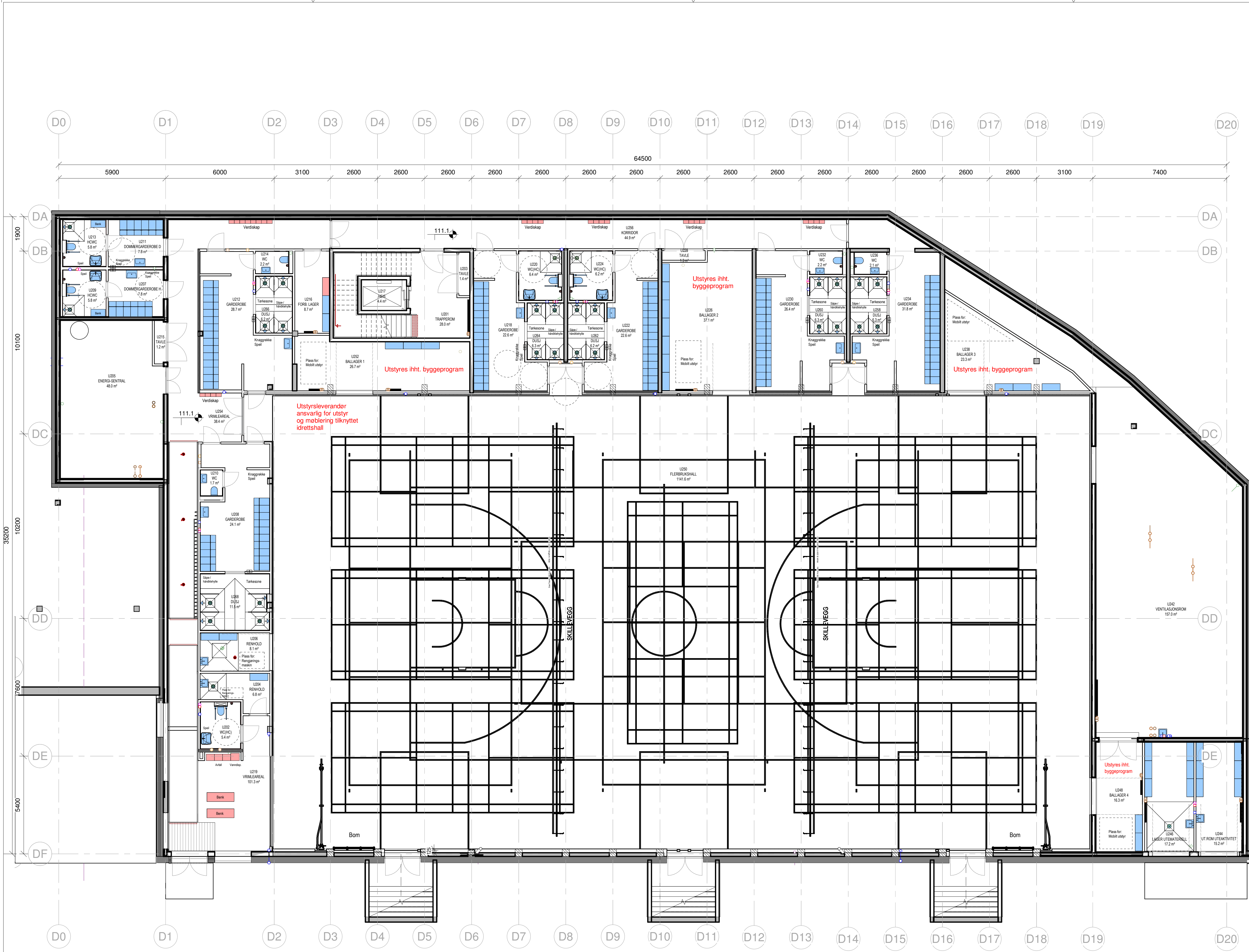
Etasje DU2_MØBLERINGSPLAN
