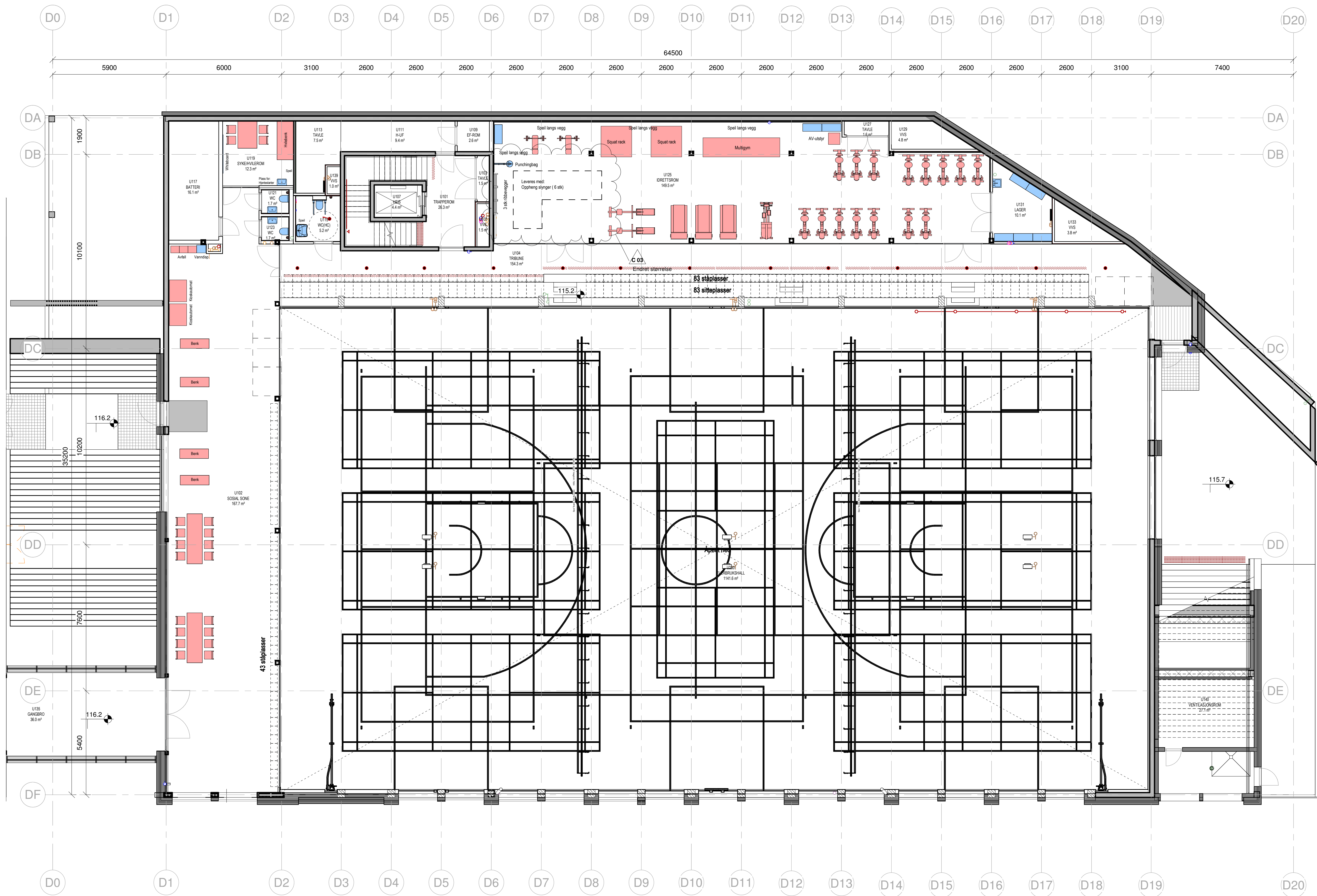
Etasje DU1_MØBLERINGSPLAN
